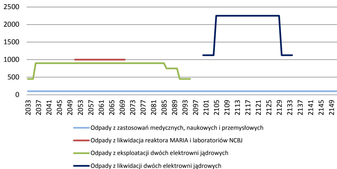
Rys. 3.5. Prognoza dostaw nisko- i średnioaktywnych odpadów promieniotwórczych do NSPOP w latach 2033-2152 [m 3 ]
