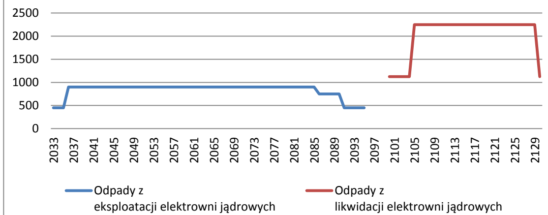
Rys.3.3. Prognoza ilości odpadów promieniotwórczych stałych nisko- i średnioaktywnych obejmująca lata 2033-2152, pochodzących z energetyki jądrowej [m 3 /rok]
